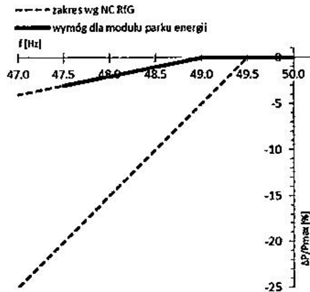
Rys. 4. Maksymalny spadek zdolności do generacji mocy przy spadku częstotliwości dla modułów parku energii
